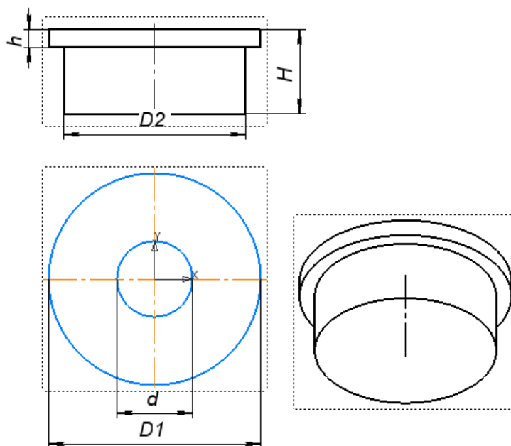
Рисунок 2.1 — Модель заглушки с размерами
